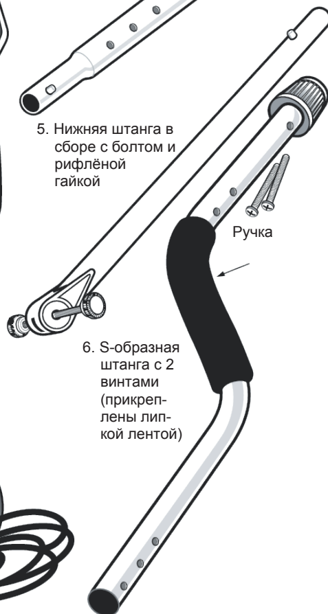
4. Средняя штанга
